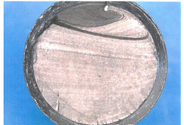
Corrosion d'un laiton au plomb.
