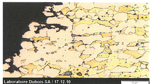
Corrosion d'un laiton au plomb.
