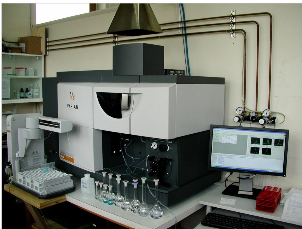
Equipement d'analyse ICP-OES
